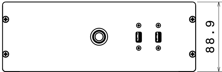
Undersicht Maßstab: 1:3
