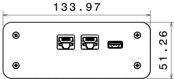
Vorderansicht Maßstab: 1:2
