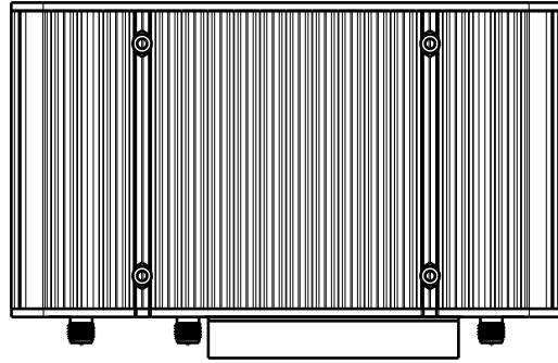
Untersicht Maßstab: 1:2
