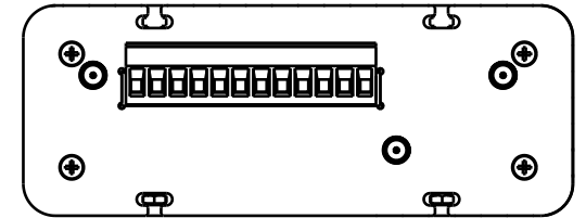
Rückansicht Maßstab: 1:2
